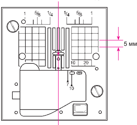
Расположение иглы по центру
